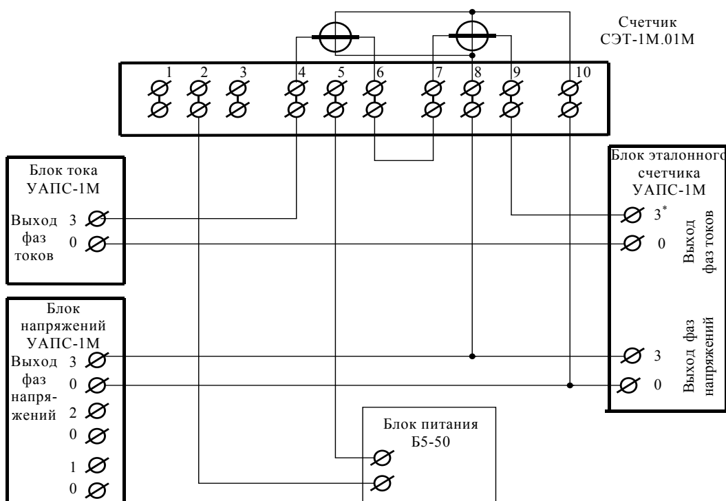
Рисунок А.2- Схема подключения счётчика к поверочной установке при раздельных цепях напряжения измерения и питания постоянного тока
